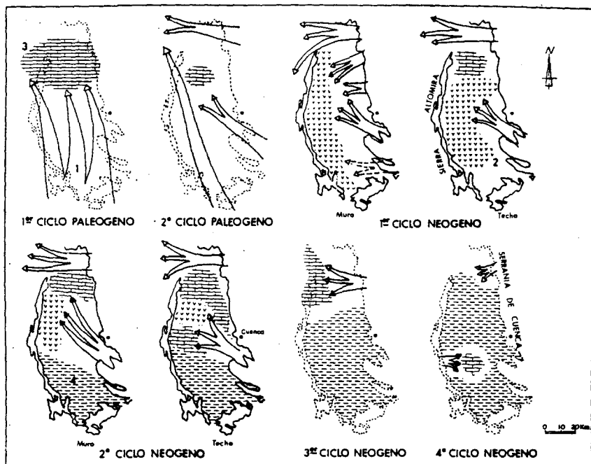
Fig. 4.3 - Evolución cenozoica de la Depresión Intermedia.
