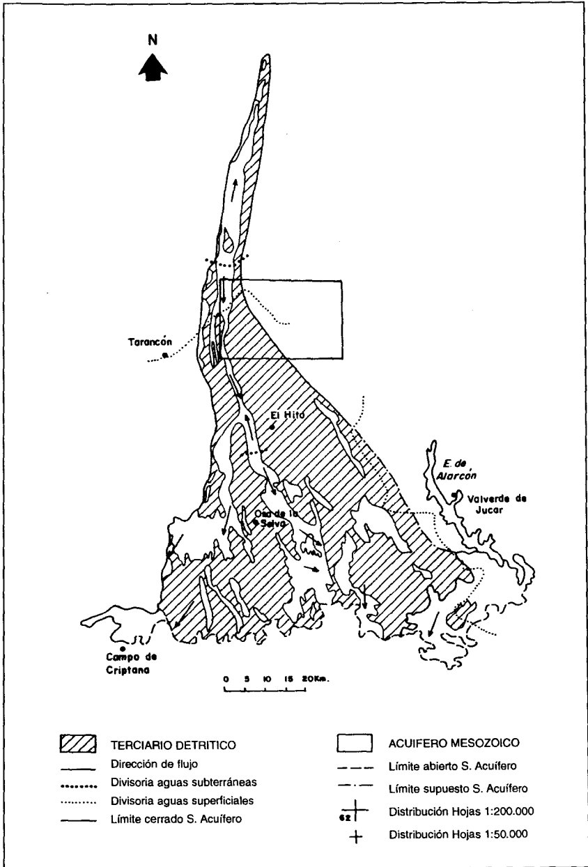
Fig. 5.3 - Sistema Acuífero: Caliza de Altomira
