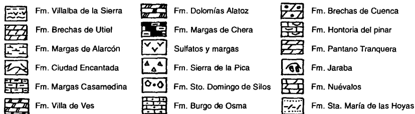
Fig. 4.2 - Evolución paleogeográfica del Cretácico superior en la Cordillera Ibérica. Depresión Intermedia y Sierra de Altomira, según MELENDEZ et al (1985).
