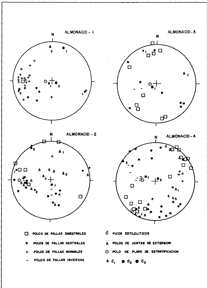
Fig. 2.2 - Proyección estereográfica equiareal de los datos de microestructuras y ejes de esfuerzo obtenidos del análisis de las estaciones Almonacid 1 (U.T.M. 30TWK 141646), Almonacid 2 (U.T.M. 30TWK 180603), Almonacid 3 (U.T.M. 30TWK154516) y Almonacid 4 (U.T.M. 30TWK138574)
