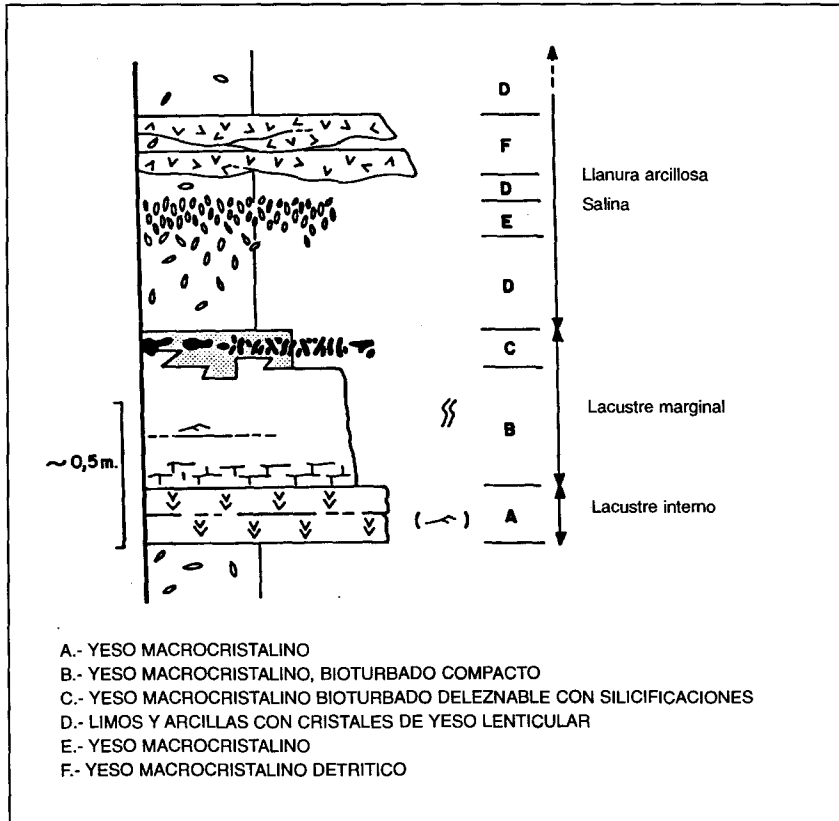
Fig. 1.7 - Asociación de facies en los sedimentos yesíferos de la "Unidad Detrítica Superior"
