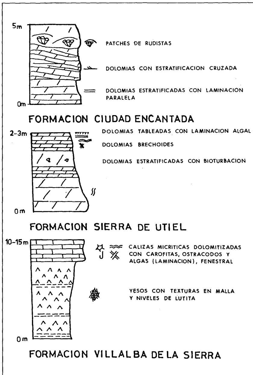
Fig. 1.3 - Secuencias elementales del Cretácico superior en la hoja de Almonacid de Zorita
