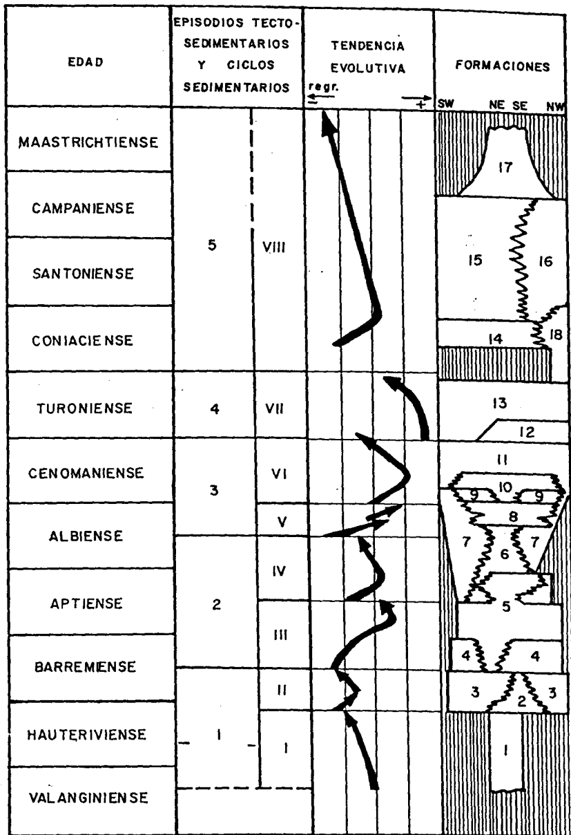
Fig. 4.1 - Ciclos sedimentarios del Cretácico en la Cordillera Ibérica suroccidental (de Vilas et al., 1982)
